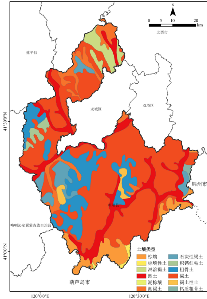
图2-10 朝阳县土壤类型分布图
