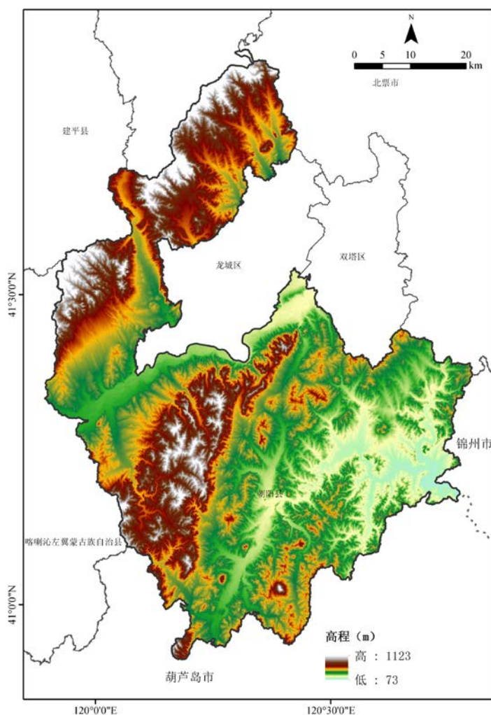
图2-7 朝阳县高程图
