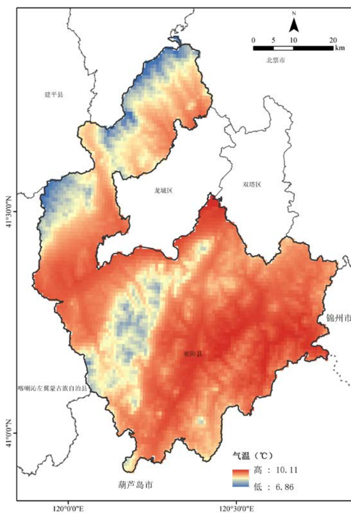
图2-8 朝阳县多年平均气温分布图
