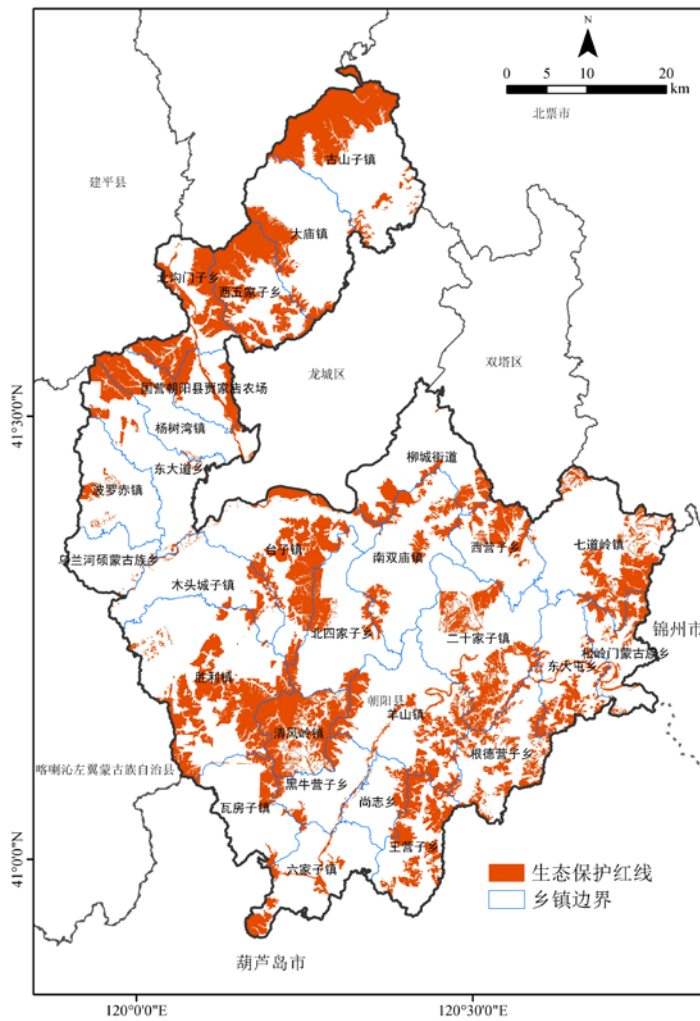
图3-1 朝阳县生态保护红线空间分布图
