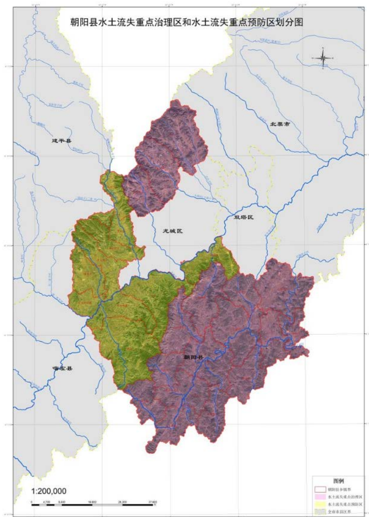
图3-2 朝阳县水土流失重点预防区和重点治理区划分图
