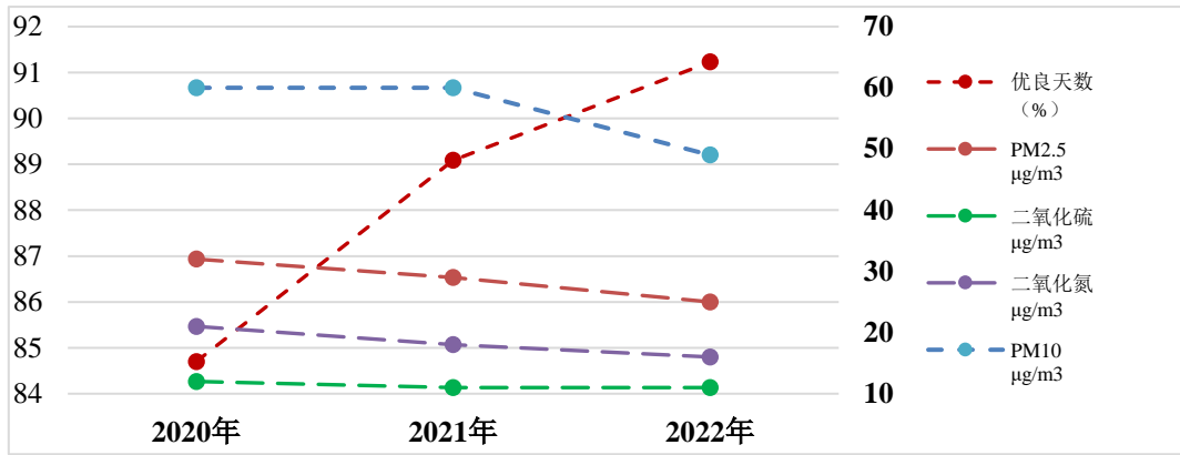
图3-3 2020-2022年朝阳县空气质量变化趋势图
