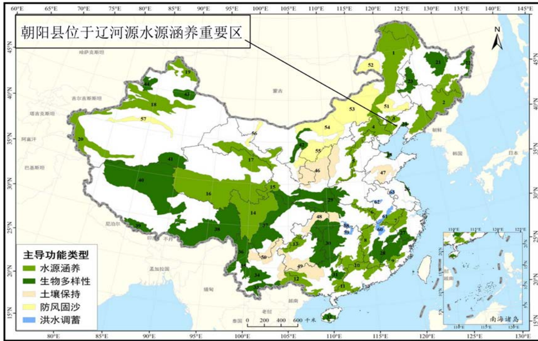
图2-4 朝阳县位于辽河源水源涵养重要区
