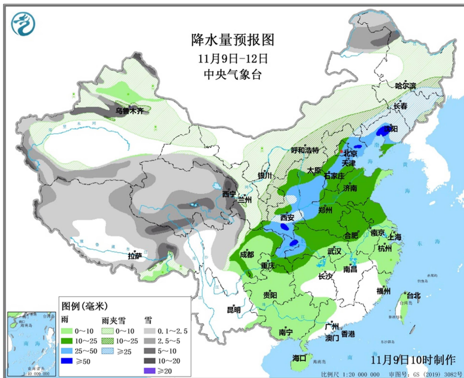
图2 降水量预报图(11月9日-12日)
