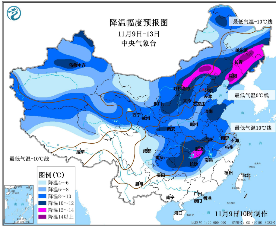
图1 降温幅度预报图(11月9日-13日)
