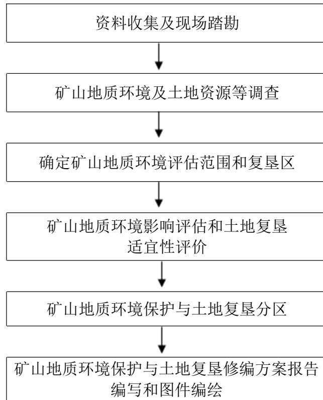
图 1 工作程序
